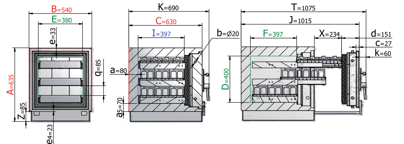
Beispiel für die Anordnung von 3 Schubladen im Oslo - Modell Art. Nr. 46500
